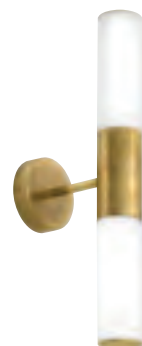
274.04.ONB 274.04.OOB 2x Max 25W G9
